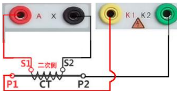
图 15 CT 变比极性电压法测试接线图
