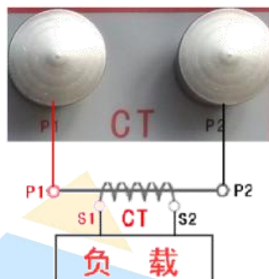
图 19 CT 一次通流接线图
