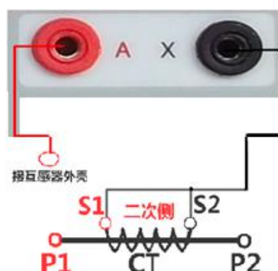
图 21 CT 交流耐压接线图
