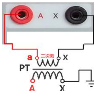
图 28 PT 励磁特性接线图
