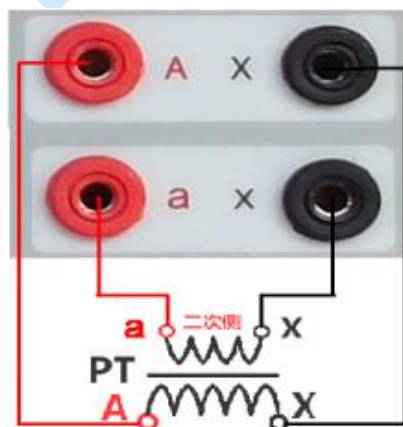
图 31 PT 变比极性 (角差比差) 接线图
