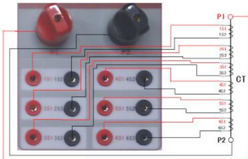
图 10 CT 变比极性（角差比差）接线图
