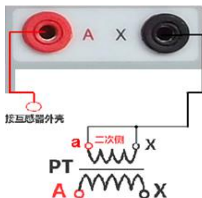
图 35 PT 交流耐压接线图
