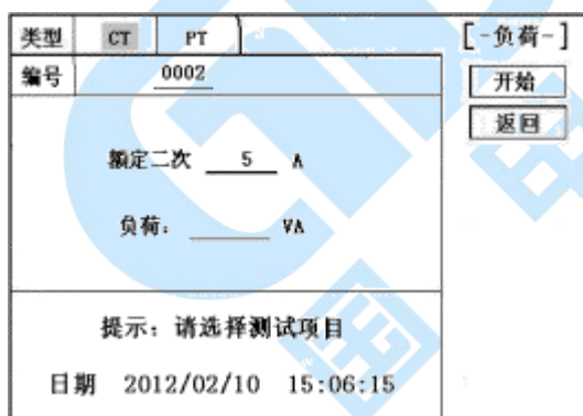
图 36 CT 二次负荷测试界面
