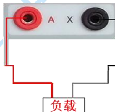
图 37 CT 二次负荷接线图
