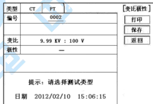
图 30 PT 变比极性测试结果界面
